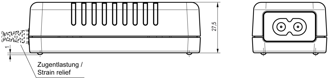
Ansicht/View A C8 Buchse/AC-Inlet
